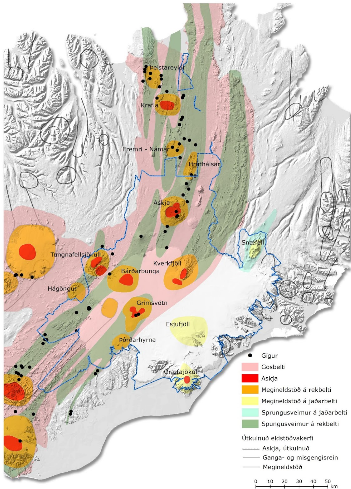
Mynd 3.6: Eldstöðvar og sprungureinar
