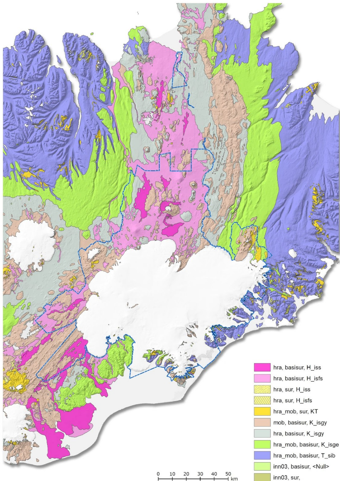
Mynd 3.5: Helstu jarðmyndanir á austurhluta Íslands.
