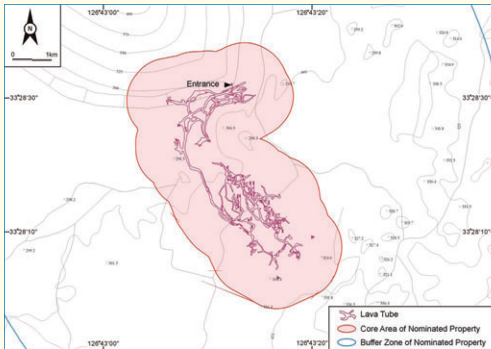
Fig. Ap.1-3-1. Bengdwigul Lava Tube plan
